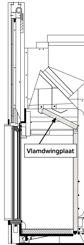
Figuur 26: W60/51F, W71/62F en W85/40F
