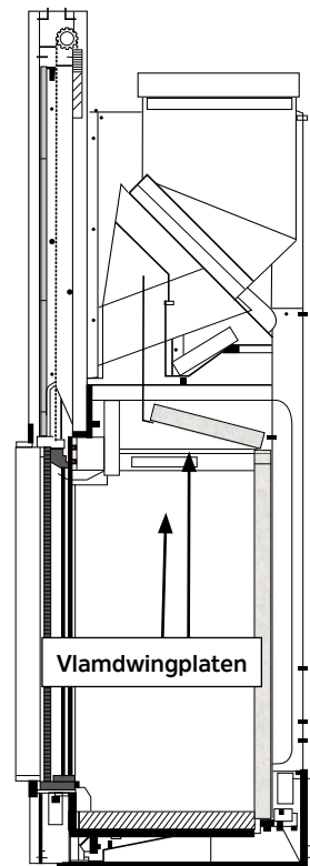
Figuur 26: W60/51F, W71/62F en W85/40F
