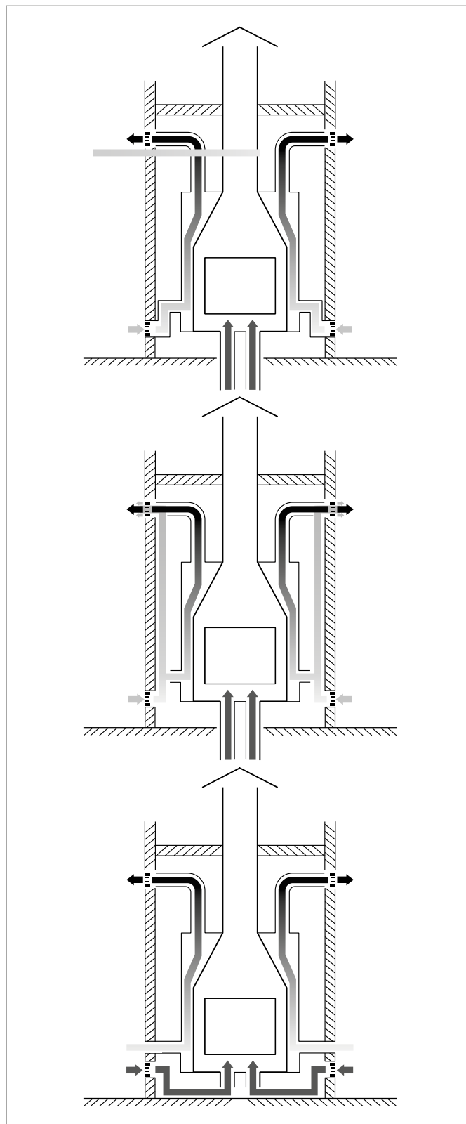
Figuur 23: Van boven naar beneden, situatie 1, 2 en 3
