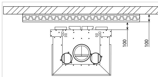
Figuur 6b: Doorsnede Kalfire W90/47S in combinatie met brandbare materialen.
