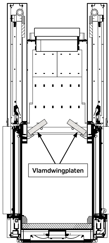
Figuur 29: W80/52T en W105/47T
