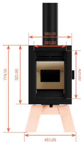
Houten voet
