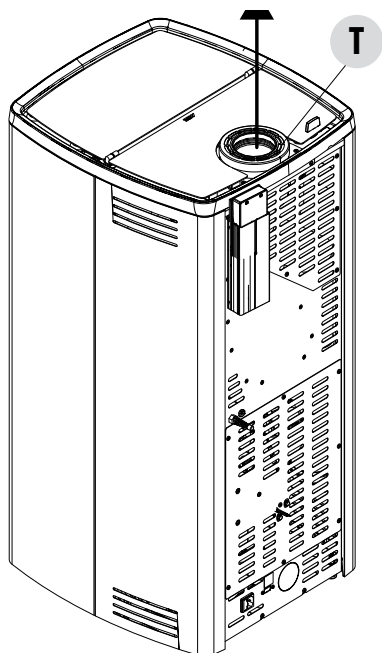
INSTALLATIE TYPE "UP" EN- KELWANDIGE ROOKUITGANG
