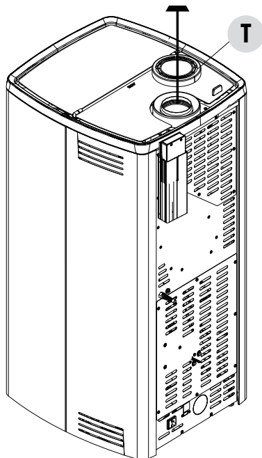
INSTALLATIE TYPE "XUP" DUBBELWAN- DIGE ROOKUITGANG
