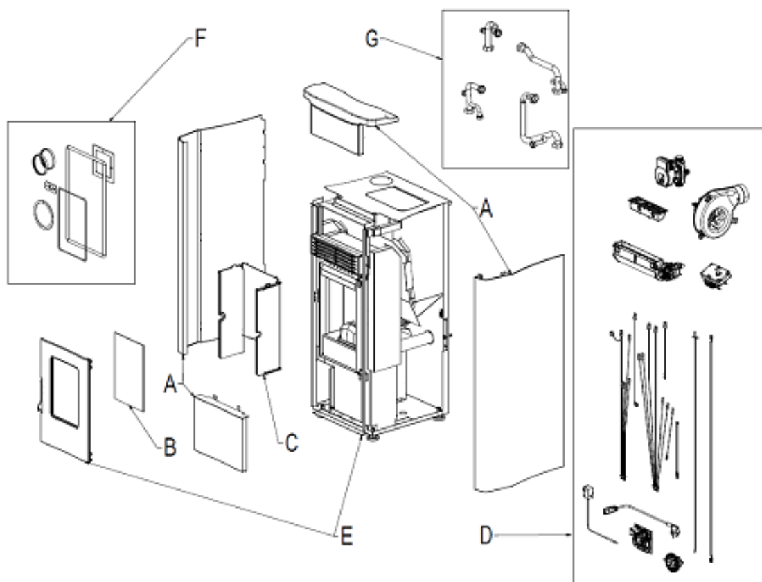
Fig. 1 - Geëxplodeerde tekening
