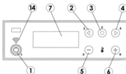
Fig. 9 - Bedieningspaneel (wi-fi)
