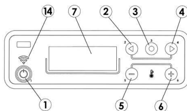
Fig. 9 - Bedieningspaneel (wi-fi)
